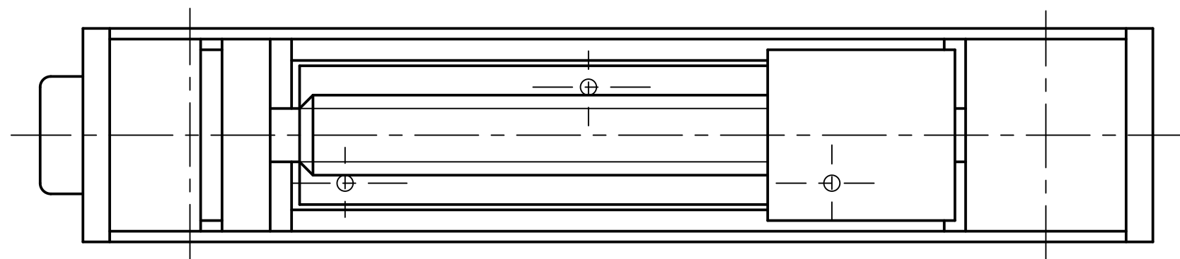
VUE DE DESSUS, RIVETS CREUX 11 ET CAPOT 10 ENLEVES
